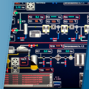
Технологічна схема САК «Станція газова поршнева» на замовлення УПГК
